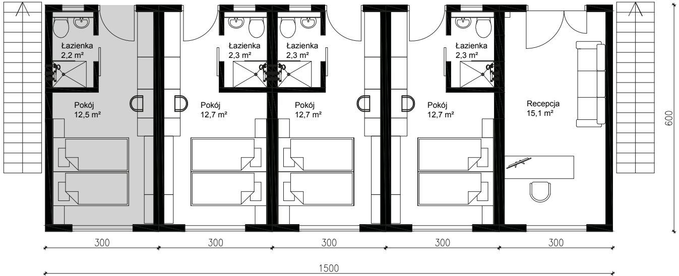
RZUT PARTERU
