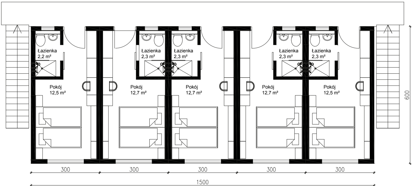
RZUT PIĘTRA
